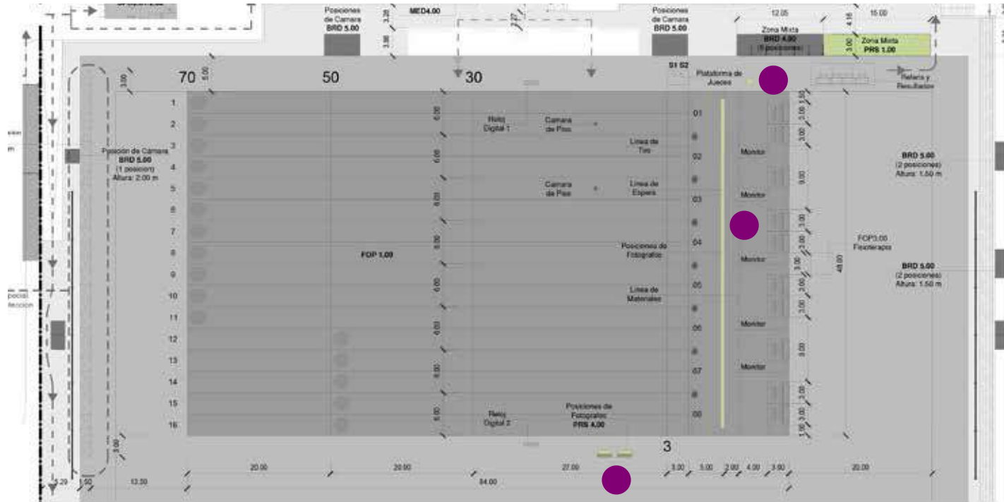
FOP TIRO CON ARCO - CAMPO SEMIFINALES ESG. 1.000
